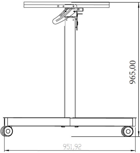
Altezza massima / Configurazione orizzontale (tavolo): 965 mm
