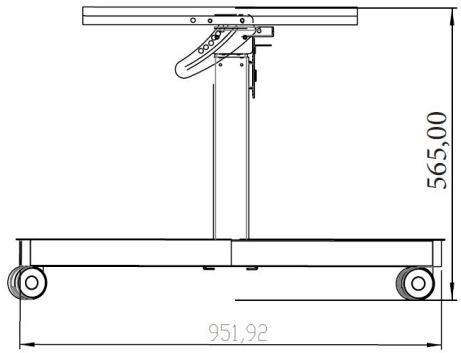
Altezza minima / Configurazione orizzontale (tavolo): 565 mm
