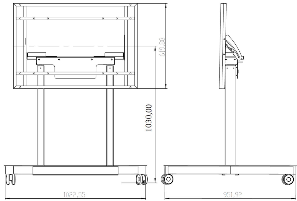
Altezza massima / Configurazione verticale: 1030 mm
