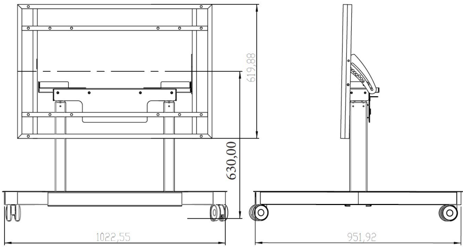
Altezza minima / Configurazione verticale: 630 mm
